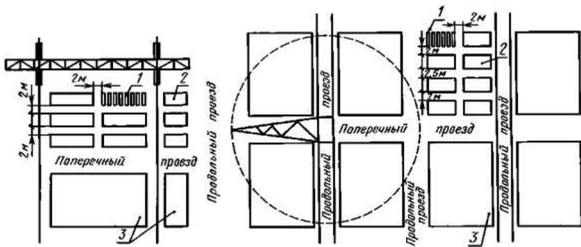
а - козловым
